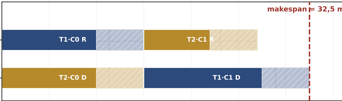
Programación óptima de carga (P2) — barra rayada = 5 min de limpieza
